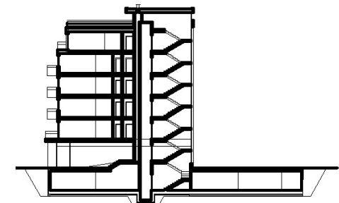
PRIEČNY REZ
