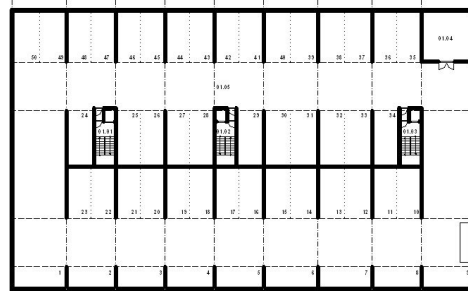
PÓDORYS 1.NP
