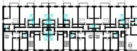
PÓDORYS 6.NP
