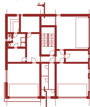
Pódorys 2.NP
