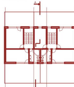
Pódorys 3.NP
