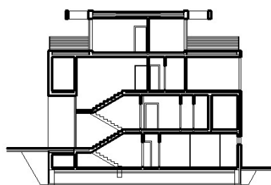
Rez A-A'
