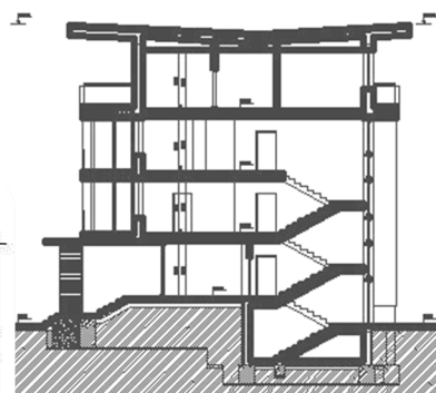
Rez A-A'
