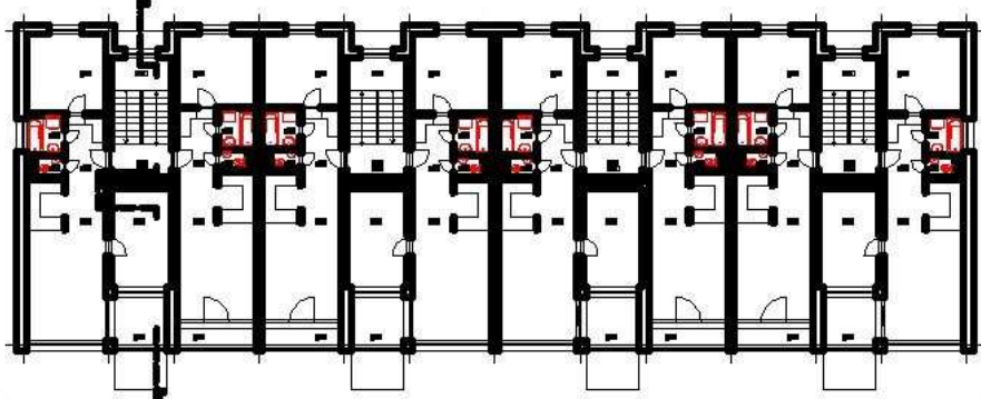
Pôdorys 2.NP
